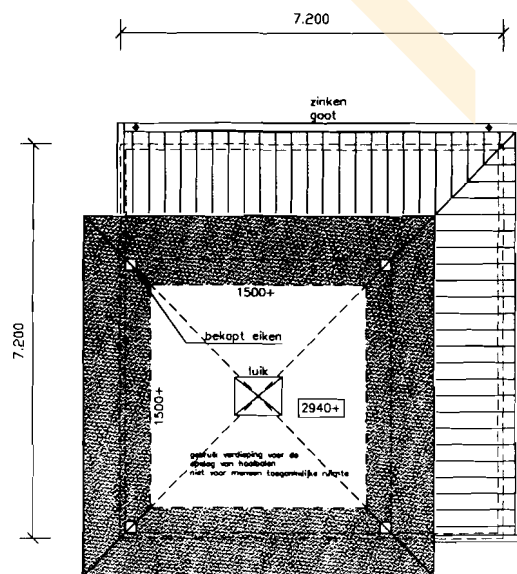
verdieping
