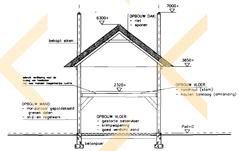
doorsnede
