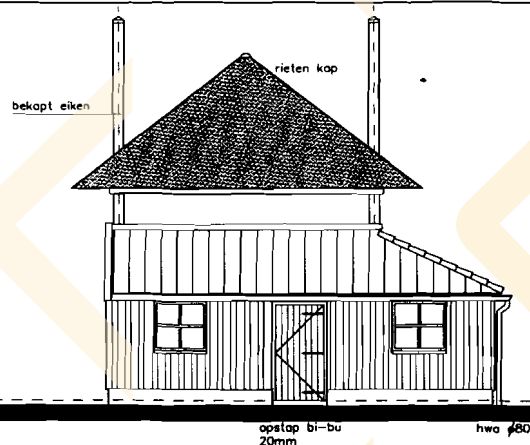
linkerzijgevel
