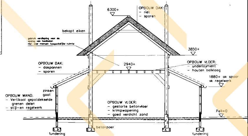
doorsnede
