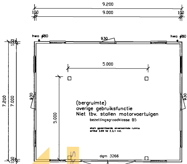
begane grond
