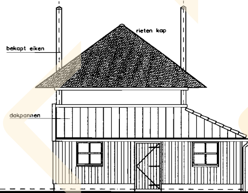
rechtzijdigevel
