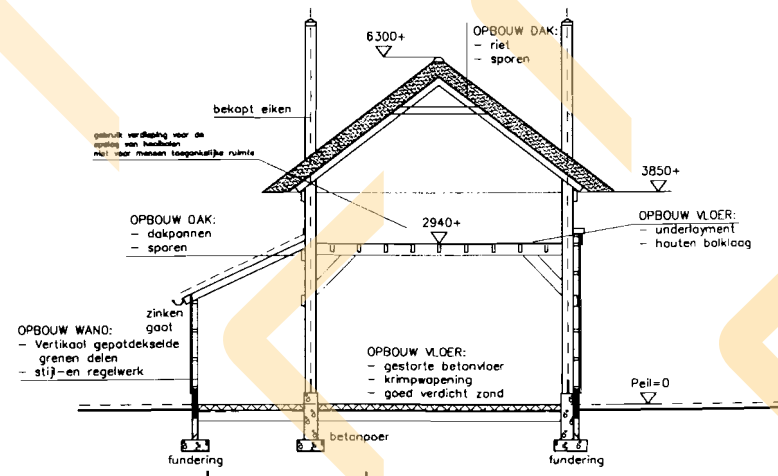
doorsnede
