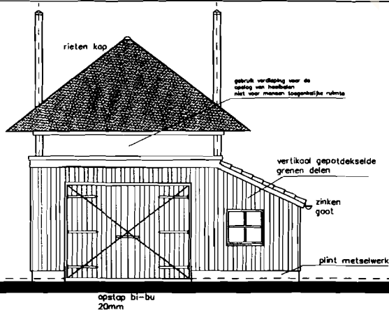
voorgevel
