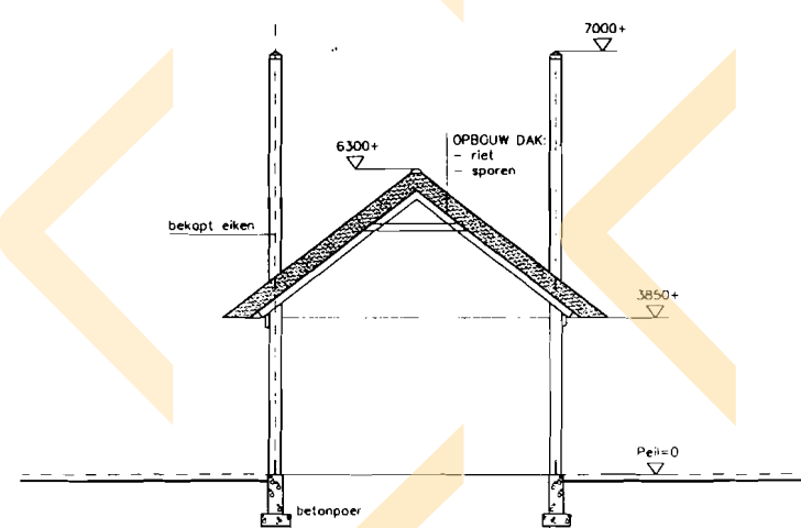
doorsnede
