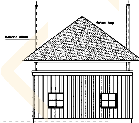
rechterzijgevel
