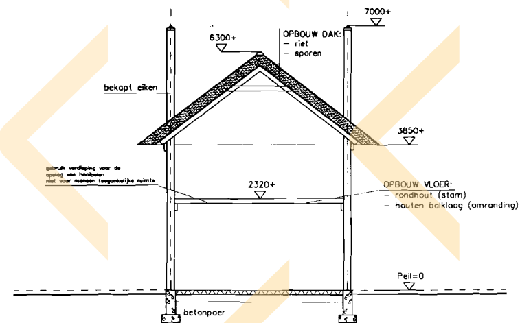
doorsnede
