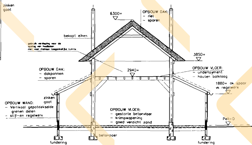
doorsnede
