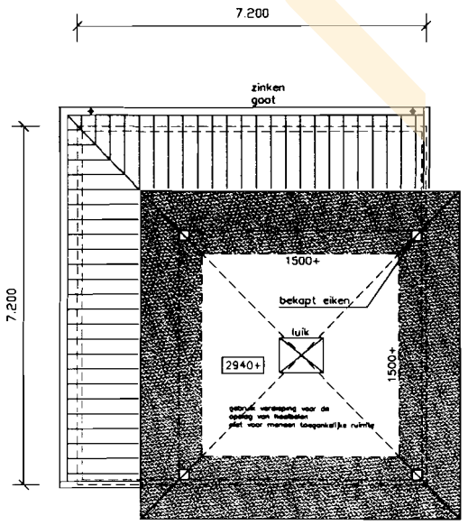
verdieping
