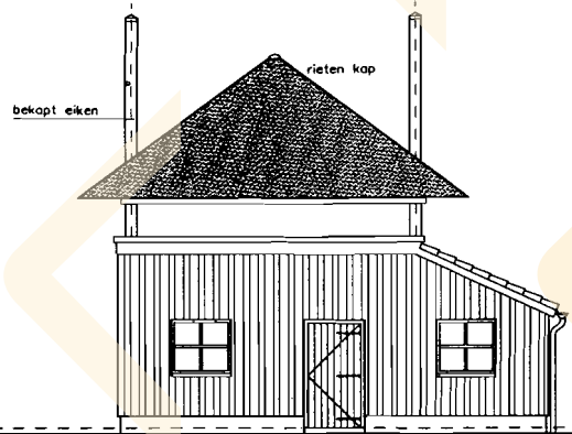
rechterzijgevel
