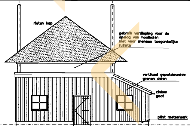
achtergevel
