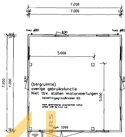
begane grond
