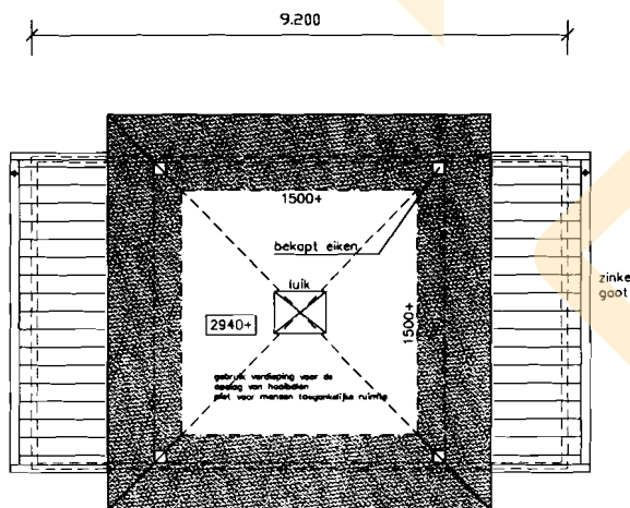
verdieping
