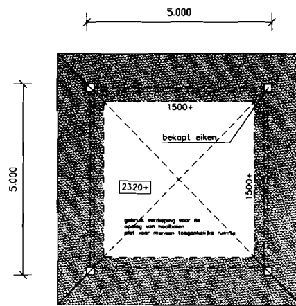
verdieping
