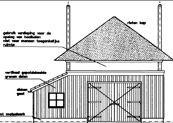
voorgevel
