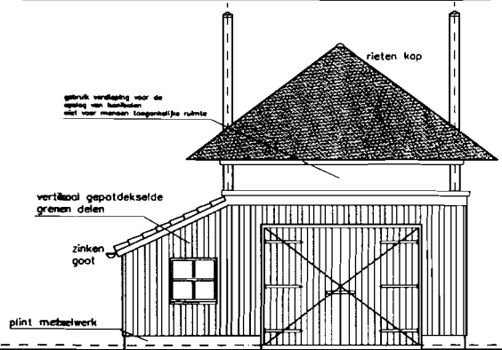
voorgevel
