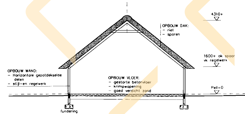
doorsnede
